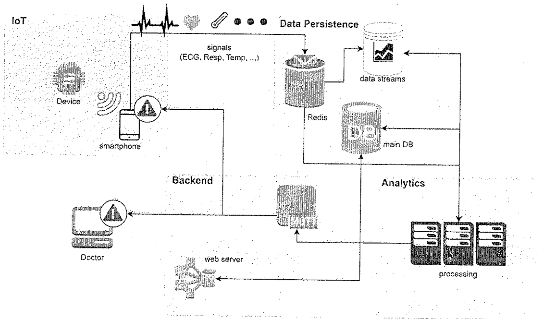
Architettura cloud della piattaforma: database, sito web e dispositivi
